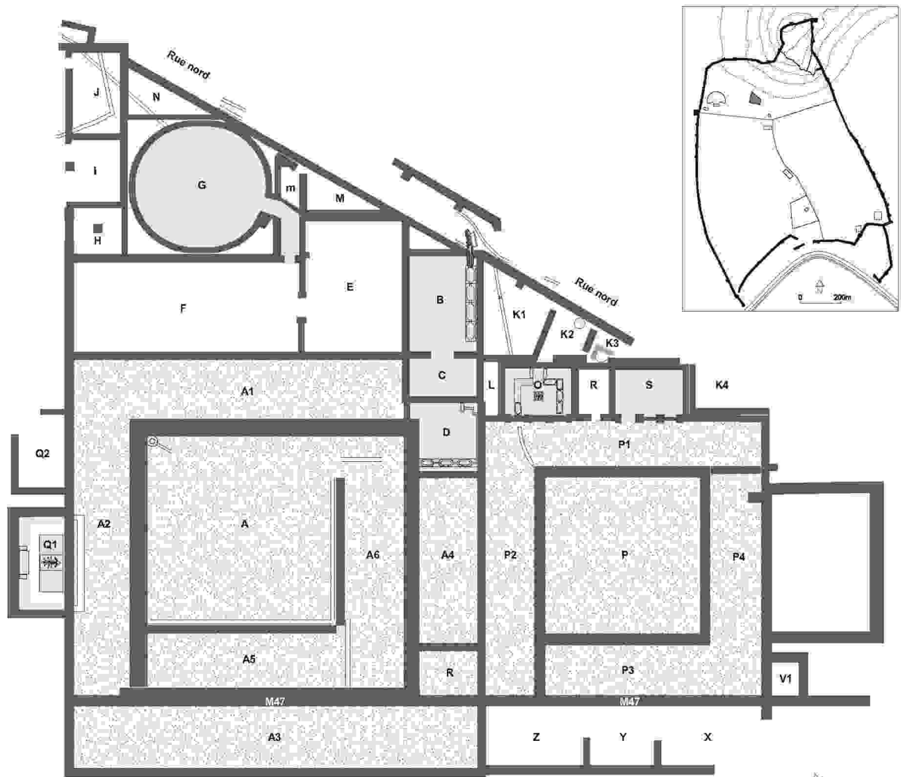
FIG. 49: Pianta del ginnasio superiore di Eretria, terza fase edilizia (150-100 a.C.) (da Ackermann et alii 2016)
