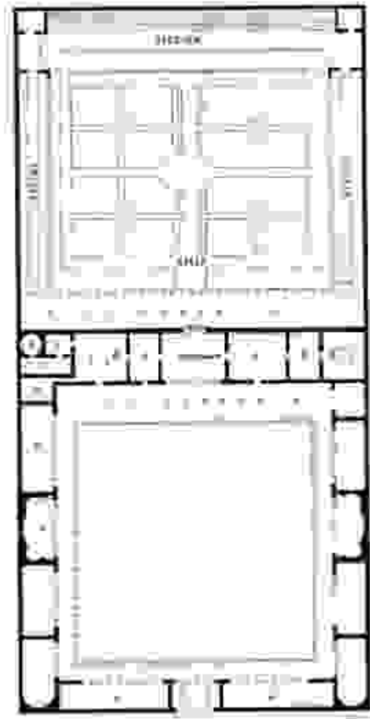
FIG. 10: ricostruzione ipotetica del ginnasio di Vitruvio (da Yegul 1992)
