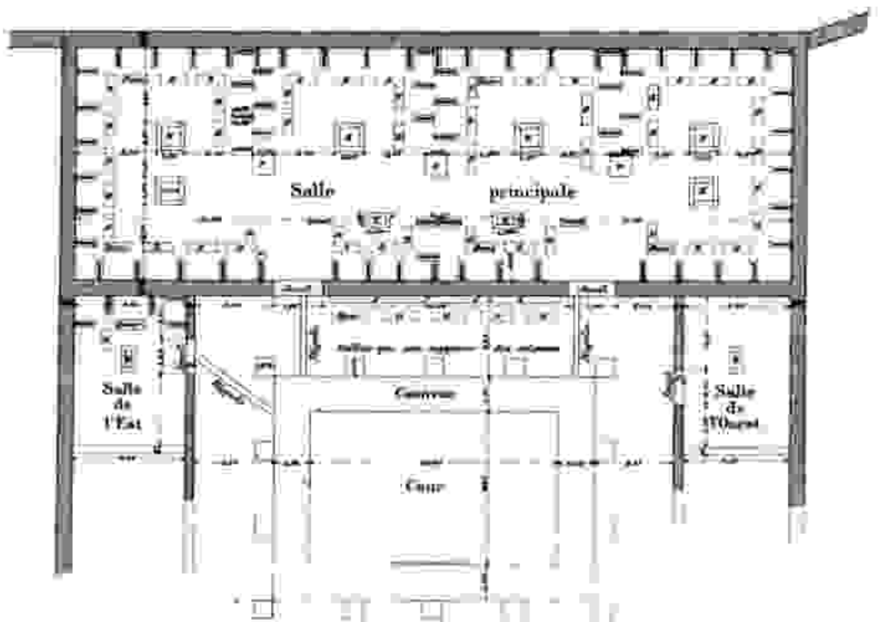
FIG. 26: pianta dell'edificio di Trezene al momento dello scavo (da Legrand 1987)
