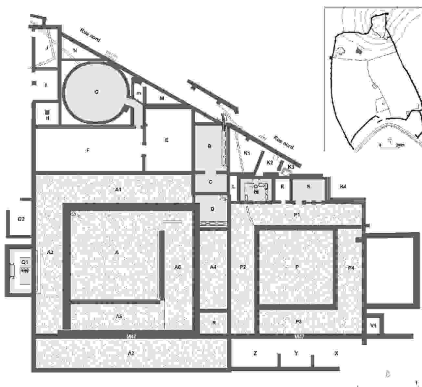
FIG 8: pianta del ginnasio superiore di Eretria; a N, gli ambienti E (sala da banchetto) e M (cucina) (da Ackermann et alii 2016)
