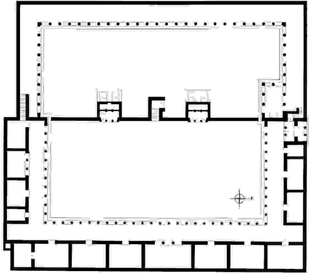
FIG. 42: Pianta e ipotesi ricostruttiva dell'alzato del ginnasio di Sicione (da Kazakidi 2012).
